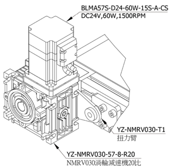
B視圖
