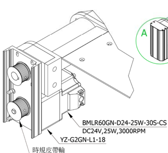
A視圖
